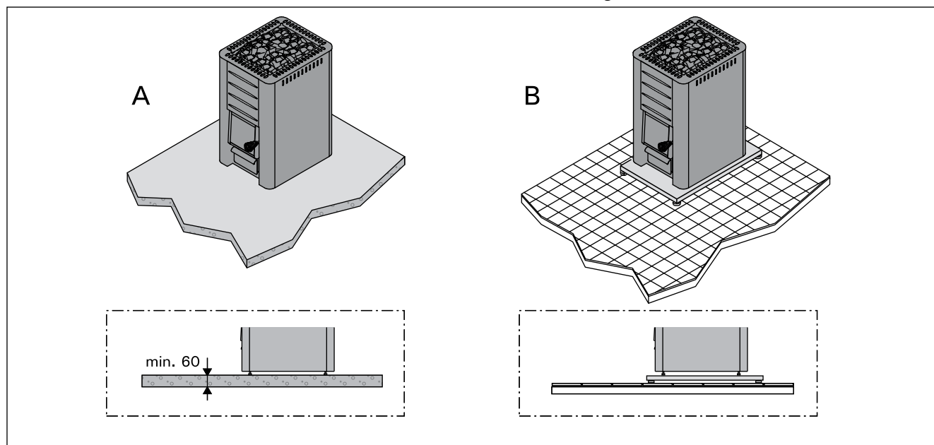
Obrázek 6. Ochrana podlahy (všechny rozměry jsou uvedeny v milimetrech) Figuur 6. De vloer beschermen (alle afmetingen in millimeters)
