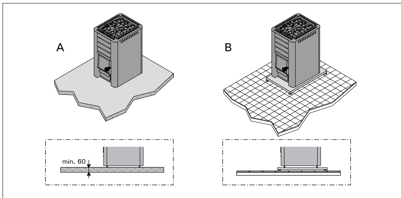
Kuva 6. Lattian suojaaminen (mitat millimetreinä) Bild 6. Skydd av golvet (måtten i millimeter)
