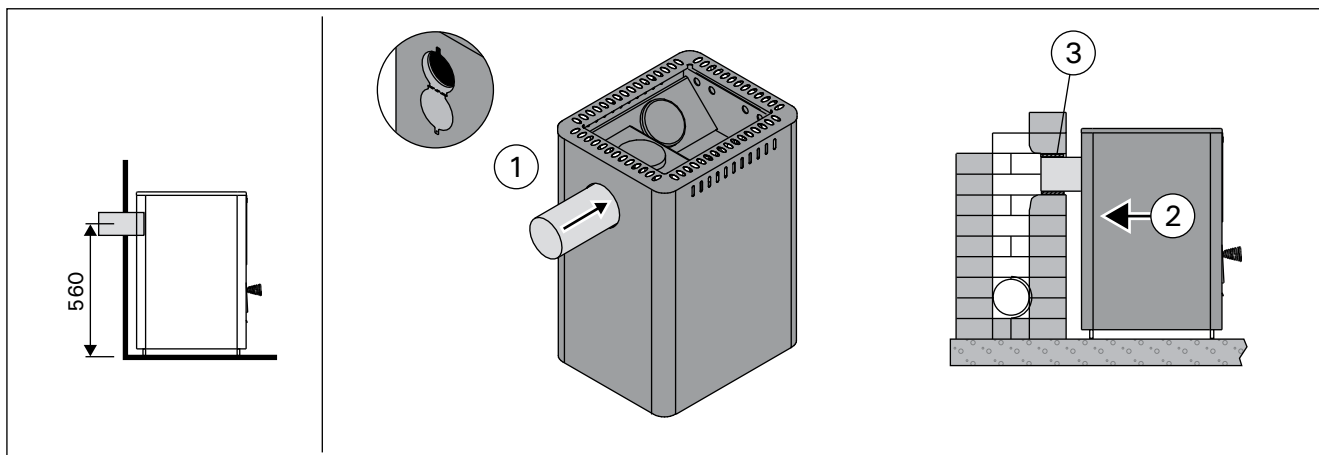
Obrázek 9. Připojení kamen k zděři ve zdi ze zadního otvoru (všechny rozměry jsou uvedené v milimetrech) Figuur 9. De kachel aansluiten op een gemetseld rookkanaal via de aansluitopening achter (alle afmetingen in millimeters)
