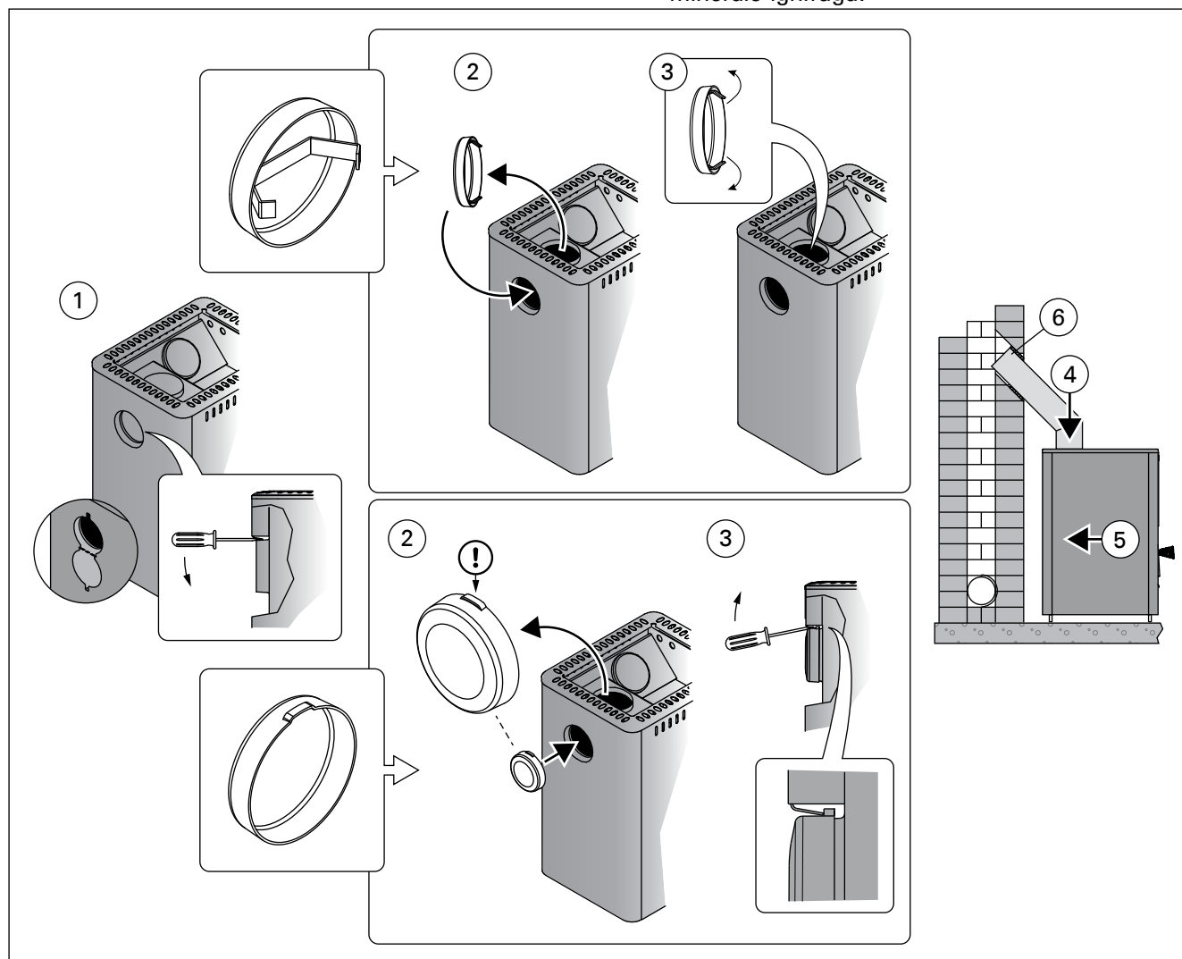
Figure 10. Raccordement du poêle à un conduit maçonné via l'ouverture de raccordement supérieure (toutes les dimensions sont fournies en millimètres)
