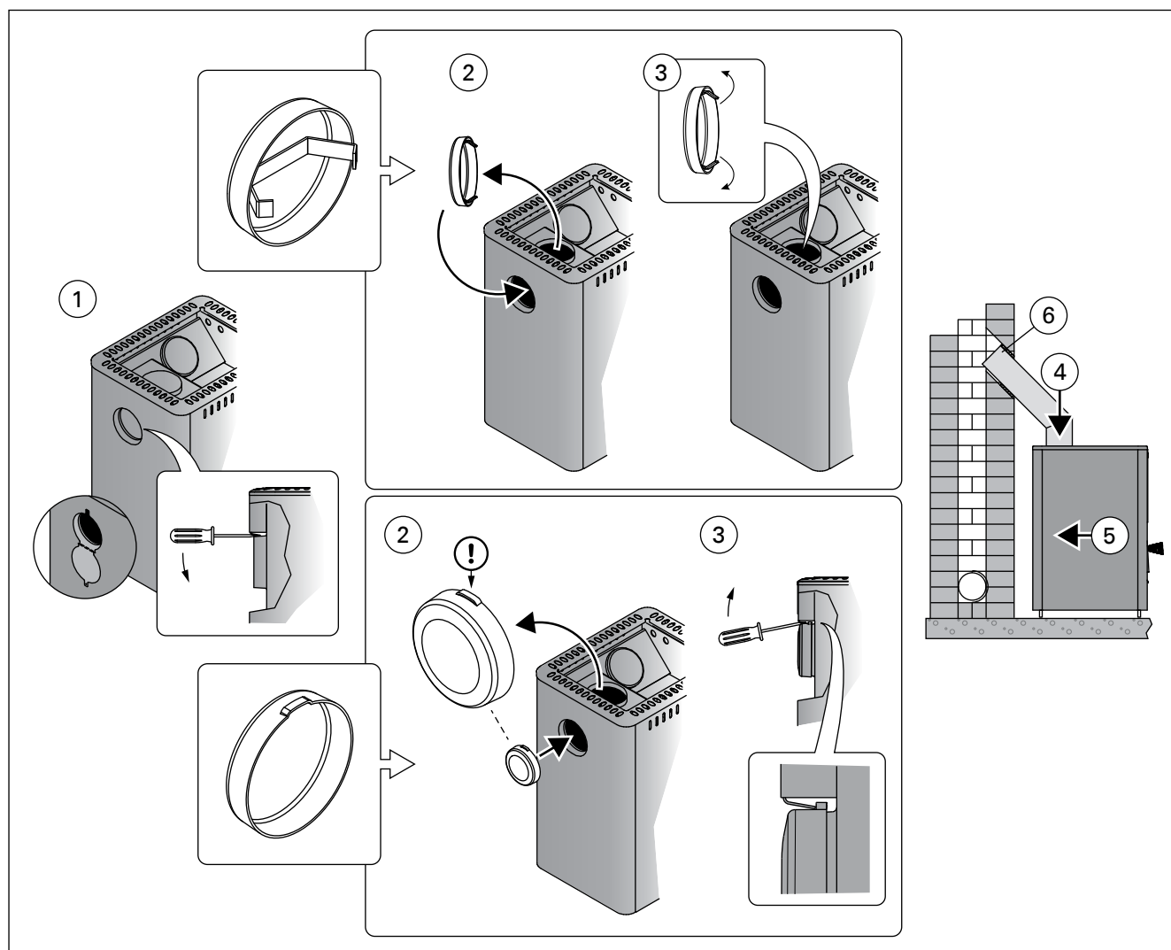
Obrázek 10. Připojení kamen ke zděři ve zdi z horního otvoru (všechny rozměry jsou uvedené v milimetrech) Figuur 10. De kachel aansluiten op een gemetseld rookkanaal via de aansluitopening boven (alle afmetingen in millimeters)
