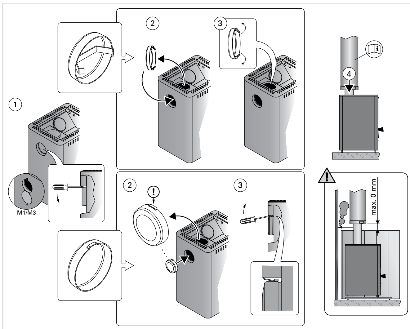
Figure 11. Raccordement du poêle à une cheminée en acier Harvia (toutes les dimensions sont fournies en millimètres) Figura 11. Collegare la stufa a una cappa in acciaio Harvia (tutte le dimensioni sono espresse in millimetri)
