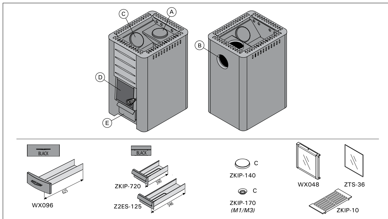
Obrázek 1. Součásti kamen. UPOZORNĚNÍ! Používejte výhradně náhradní díly doporučené výrobcem. Neoprávněné úpravy kamen jsou zakázány.
