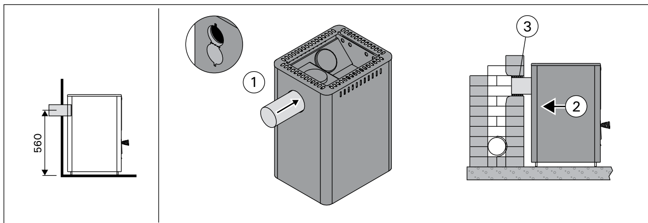
Figure 9. Raccordement du poêle à un conduit maçonné via l'ouverture de raccordement arrière (toutes les dimensions sont fournies en millimètres)
