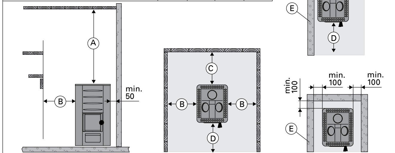
Obrázek 7. Bezpečné vzdálenosti pro topné těleso (všechny rozměry jsou uvedené v milimetrech) Figuur 7. Veiligheidsafstanden (alle afmetingen in millimeters)
