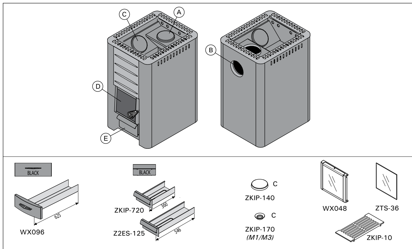
Figure 1. Composants du poêle. Note! Utilisez uniquement les pièces de rechange recommandées par le fabricant. Toute modification du poêle sans autorisation est interdite.
